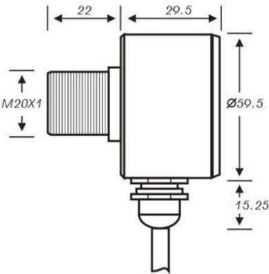
图 5-1b 外型尺寸
