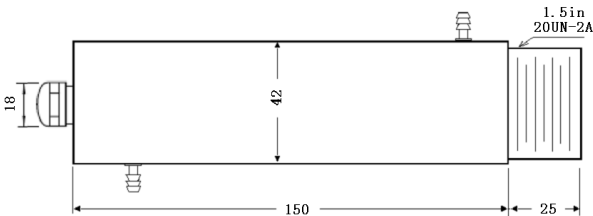
图 5-1b 外型尺寸
